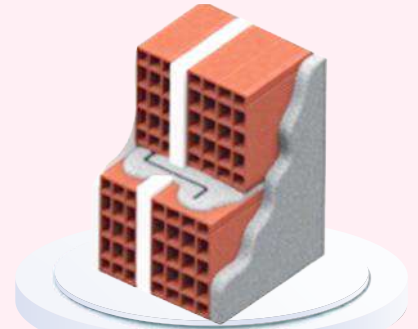
Z Metalli Sandviç Tuğla Duvar
